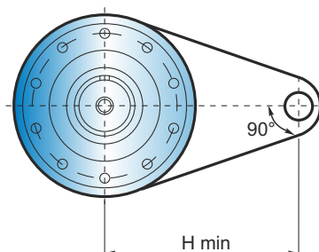
Abbildung 10: Drehmomentenstütze
