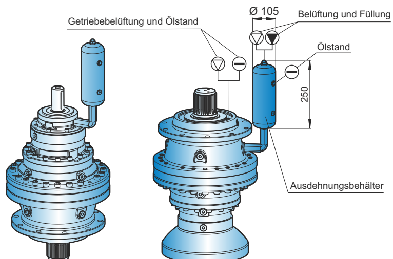
Abbildung 8: Ausdehnungsbehälter
